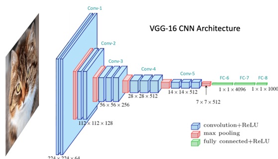
Figura 2.4: Estructura clásica de las CNN. Fuente (?).
