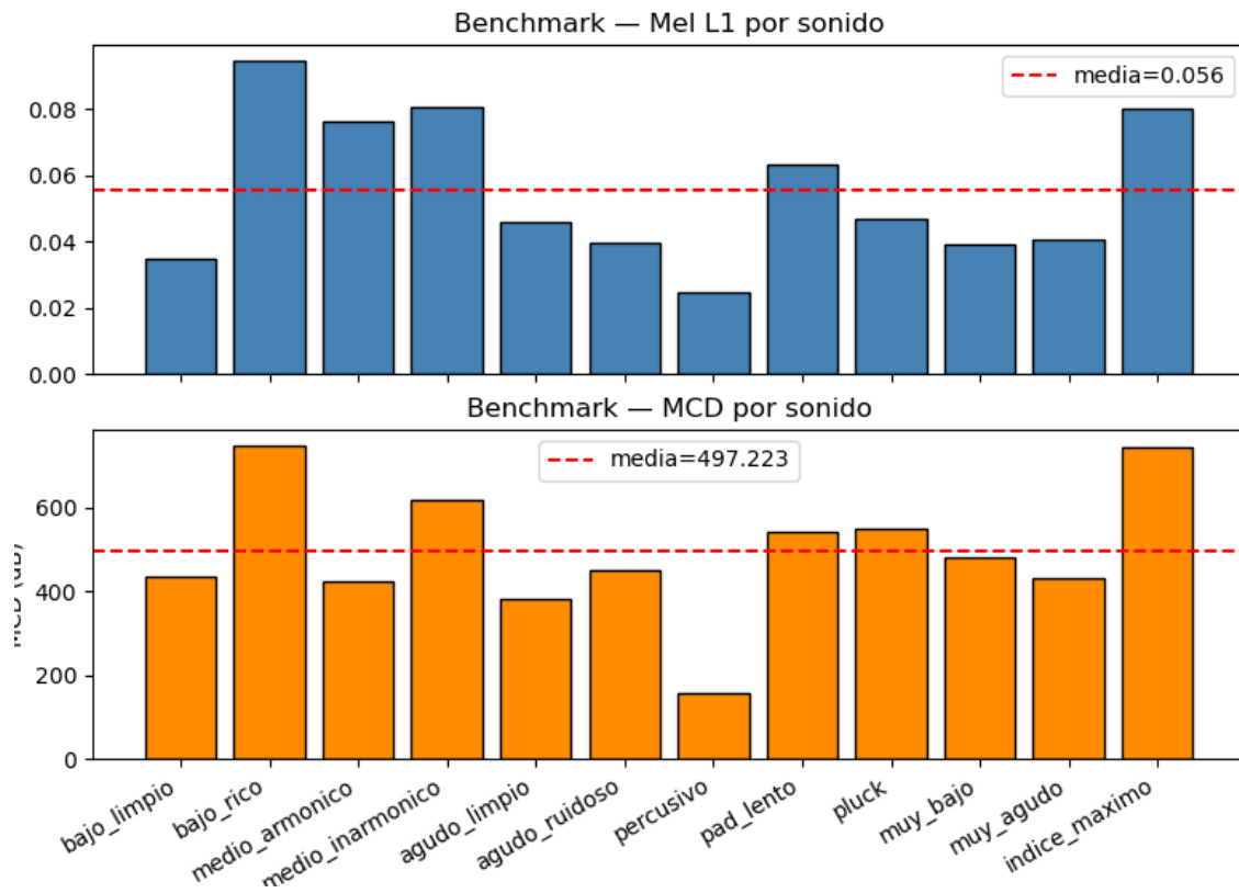
Figura 5.7: Gráfico obtenido en la evaluación de P4 mediante benchmark .
