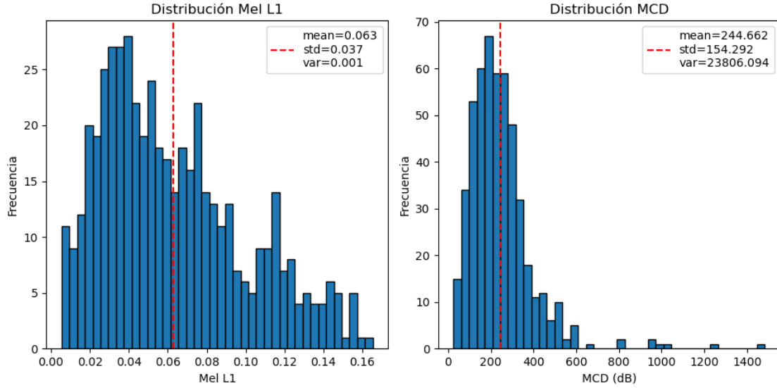
Figura 5.2: Graficas que muestran los resultados de evaluar el conjunto de tests sobre el modelo P2 con las métricas Mel L1 y MCD.
