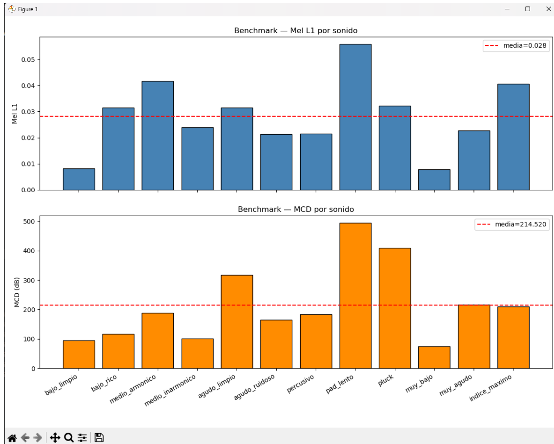
Figura 5.3: Gráfico obtenido en la evaluación de P2 mediante benchmark .
