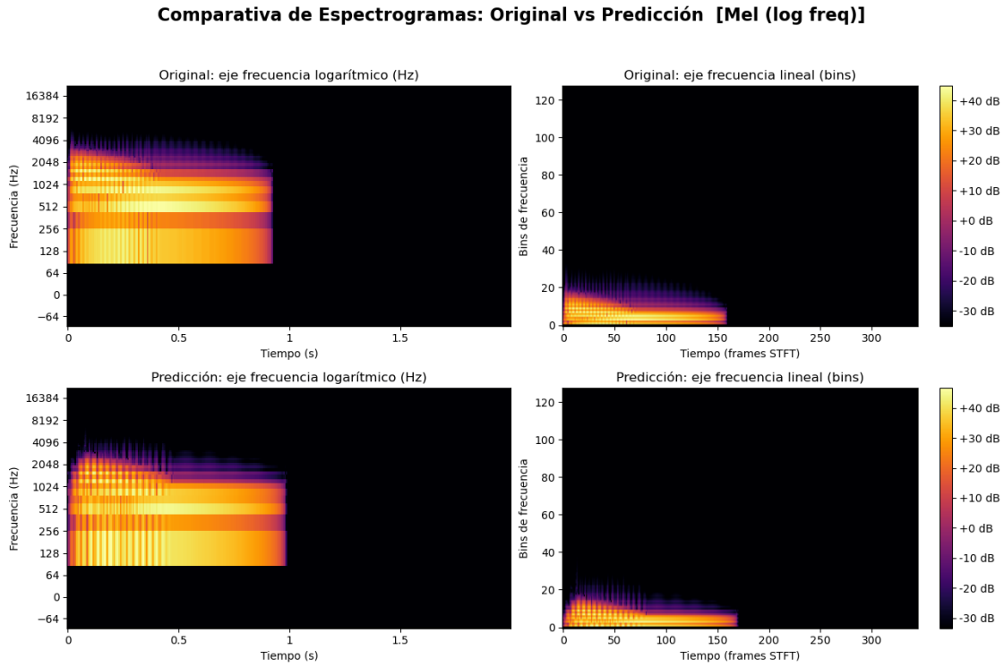
Figura 5.4: Espectrograma resultado de la predicción del audio de Benchmark: muy_bajo .
