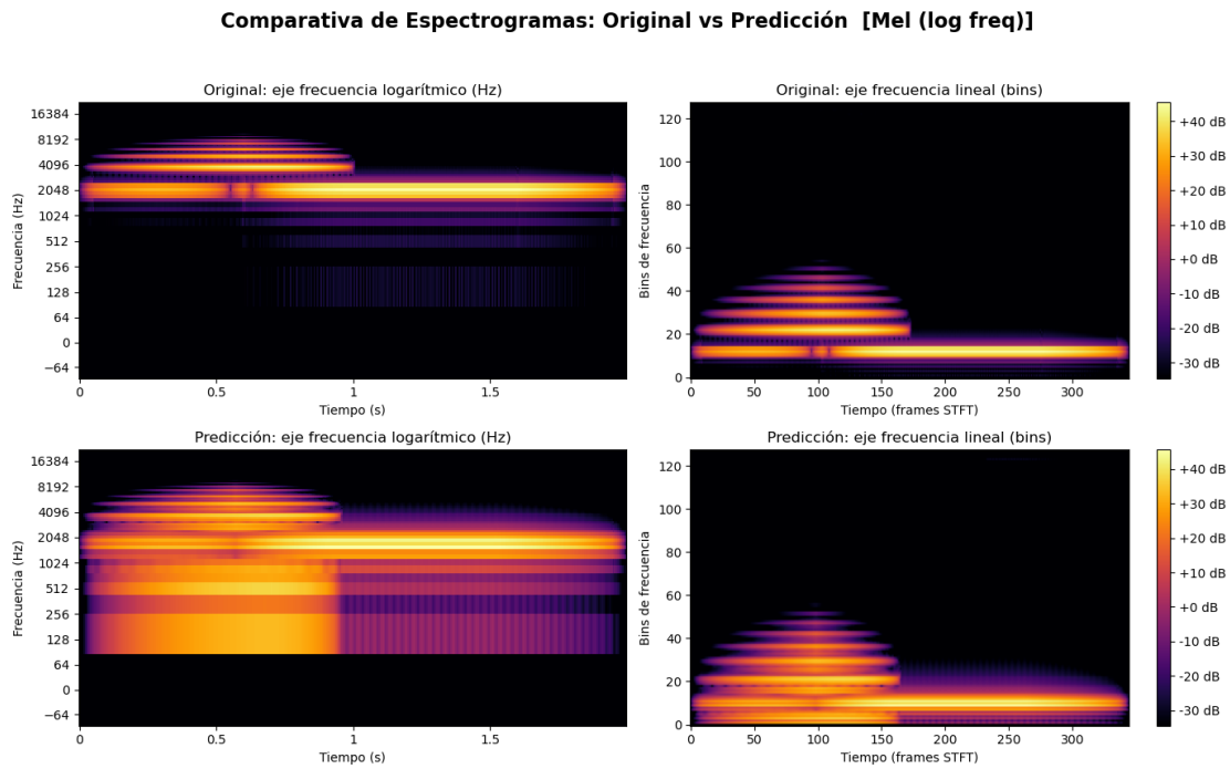
Figura 5.5: Espectrograma resultado de la predicción del audio de Benchmark: pad_lento .
